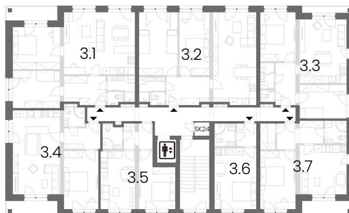
Půdorys 3.NP
