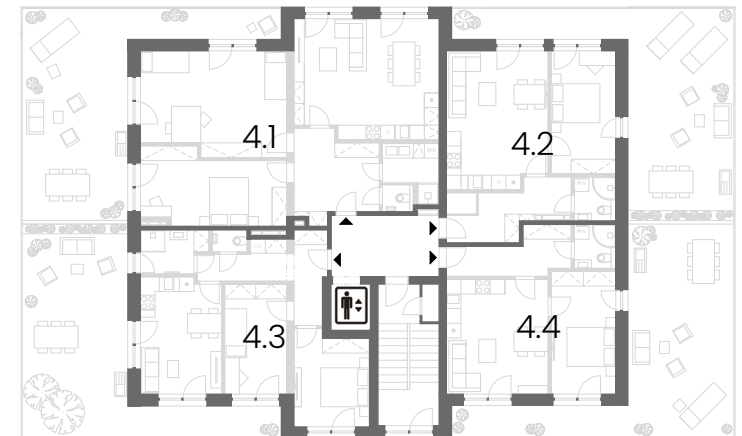
Půdorys 4.NP
